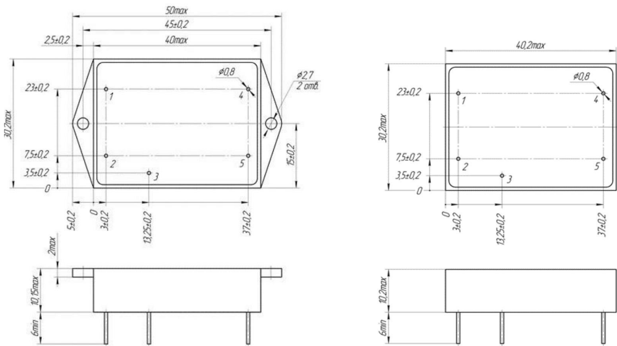
Исполнение с фланцами (индекс “У”)
